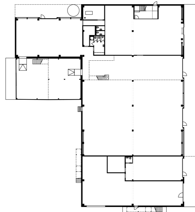
Grundriss Erdgeschoss
